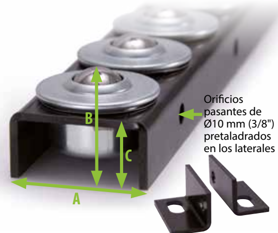
Escuadras de fijación RB-1 (a ambos lados)
